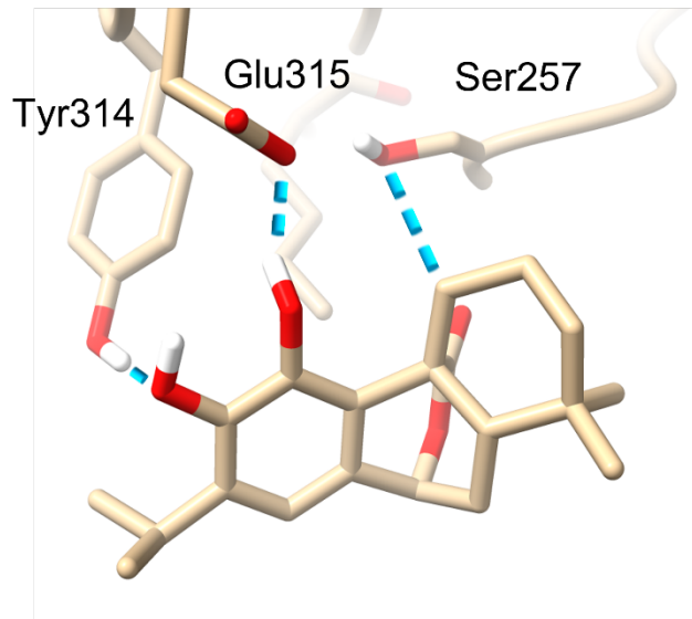
carnosol
