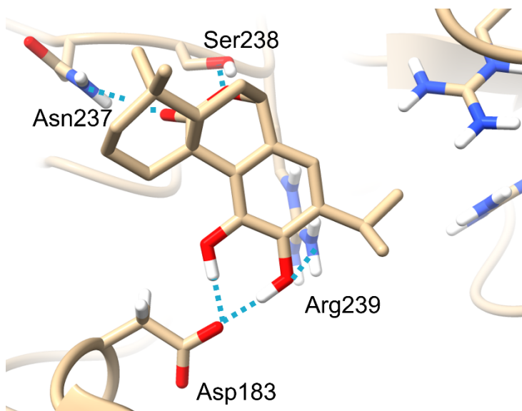
carnosol
