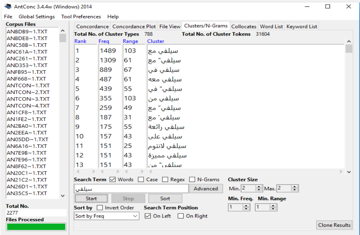
Figura 5 - Cluster Types calcolati: Rank, Frequenza, Range e Cluster.
