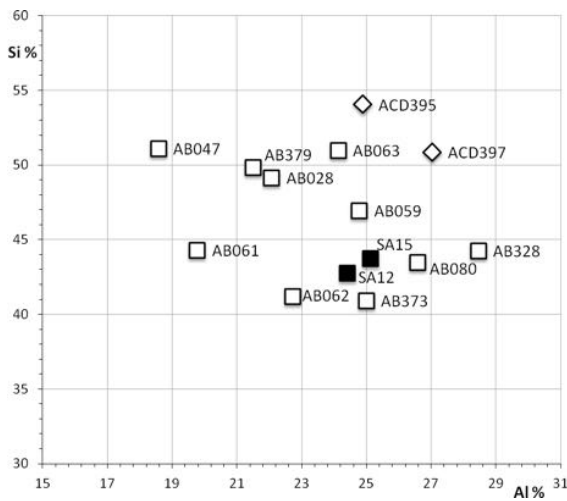
Fig. 18 : Étude archéométrique. Diagramme binaire silicium - aluminium des sigillées africaines de la collection Albert-Buès (AB), de l'atelier de Sidi Aïch (SA) et de l'atelier de Sidi Khalifa (ACD). (Analyses exprimées en %, cf. tableau 2). (J.-P. Ambrosi).
