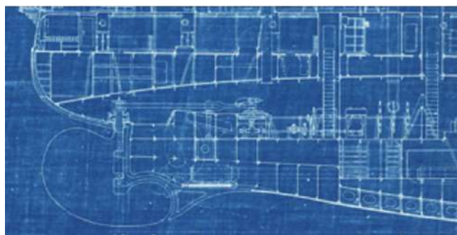
RN Regina Margherita , dettaglio poppa dal disegno vista longitudinale, Archivio DuilioShip
