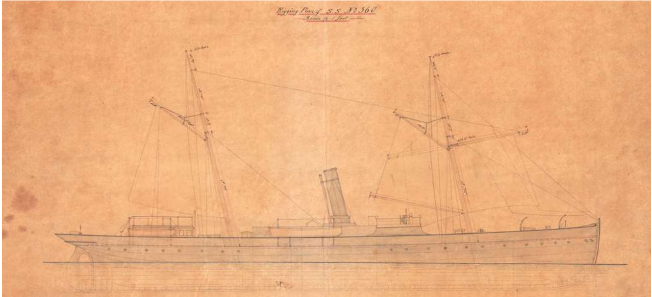
S.S. N 360 Rigging plan, china nera su lucido scuro, Archivio DuilioShip
