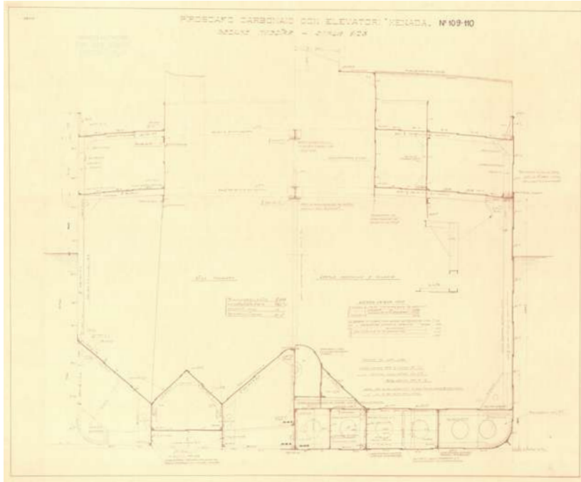
Piroscafo carbonaio con elevatori Menada, sezione maestra, cianografia seppia, Archivio DuilioShip
