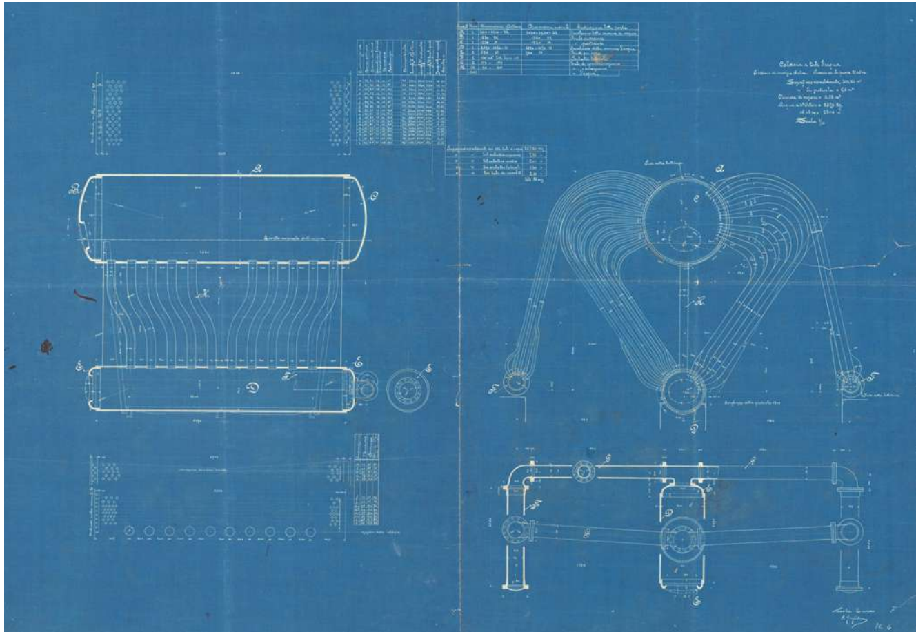
Caldia a tubi d'acqua triangolare con collettore acqua e vapore superiore e 3 collettori acqua alla base, blueprint, Archivio DuilioShip
