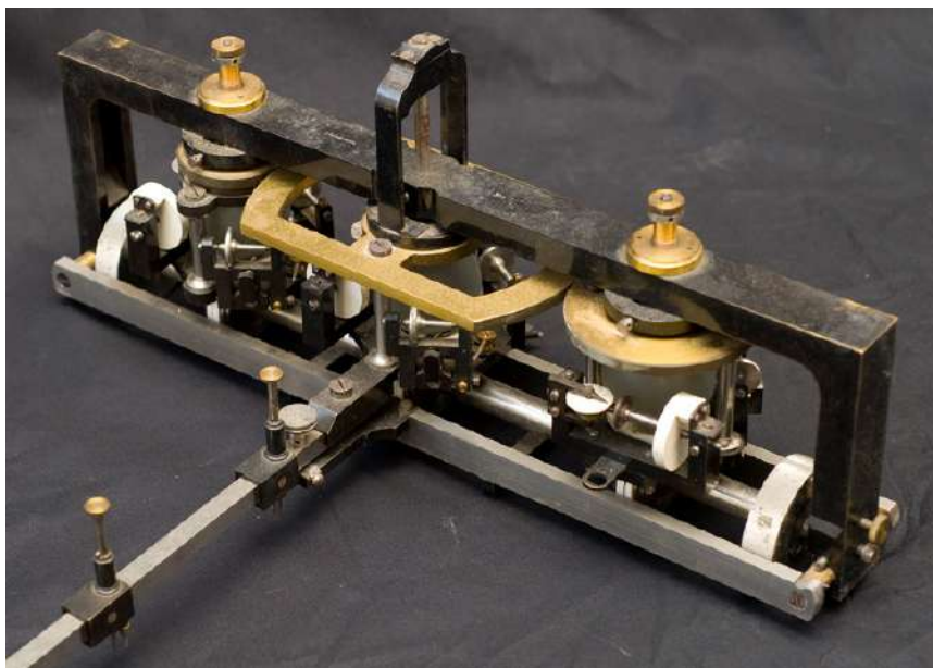
Integratore a disco su carrello e guida a rotolamento, progettato dal prof. H.S. Hele Shaw, Liverpool, 1913. Raccolta strumenti conservati presso il DITEN
