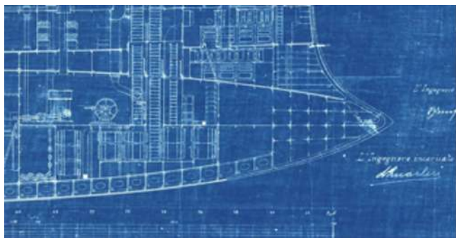
RN Regina Margherita , dettaglio prua a sperone dal disegno vista longitudinale, Archivio DuilioShip
