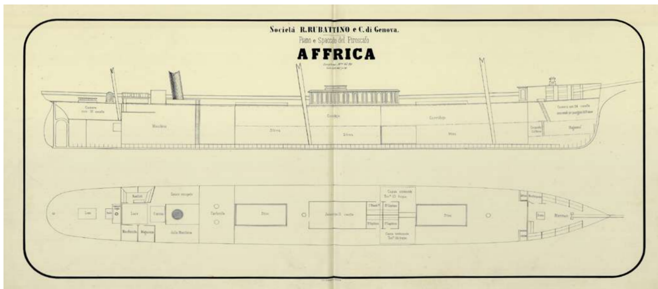
Piroscalo 'Affrica' Tavola tratta da «Materiale navale della Società R. Rubattino e C. Concessionari dei servizi postali marittimi», Archivio DuilioShip
