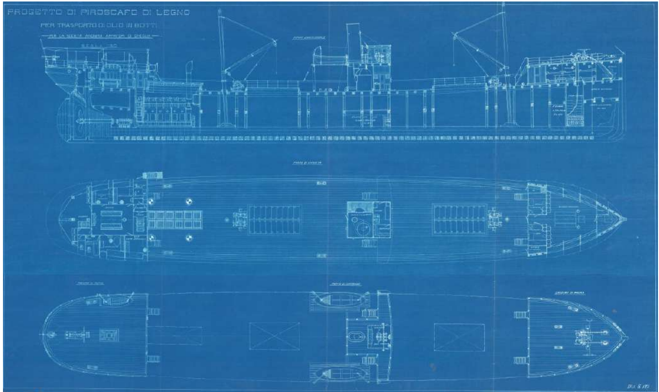
Progetto di piroscrafo per trasporto olio in botti, Piano di struttura, blue print, raccolta disegni provenienti da DITEN, Archivio DuilioShip
