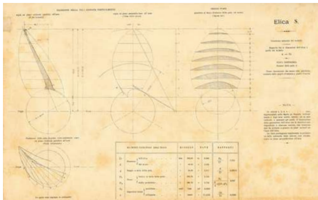
Tavola IV dell'annale. Disegno dell'elica S1 per i modelli del piroscalo Kaiser Friedrich
