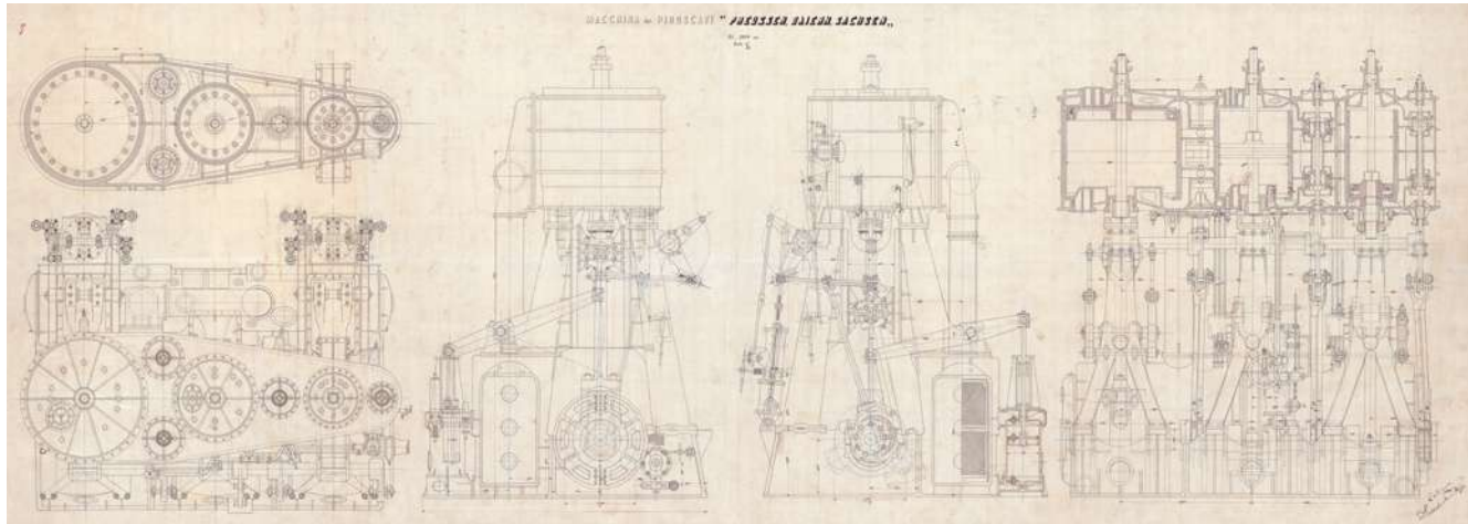
Macchina per piroscafi Preussem Baier, Sachsen, cianografia da lucido a china, Archivio DuilioShip
