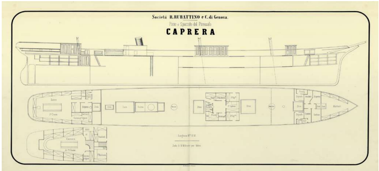
Piroscalo Caprera, particolare tratto da «Materiale navale della Società R. Rubattino e C. Concessionari dei servizi postali marittimi», Archivio DuilioShip
