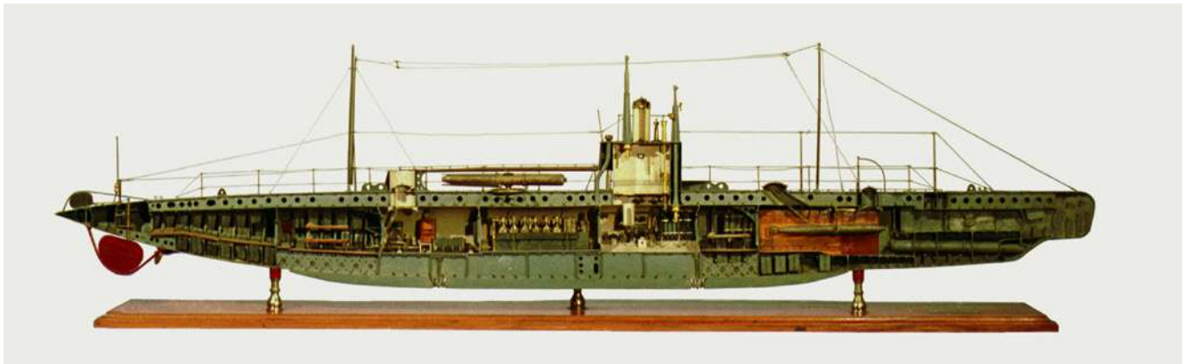
Sommersibile torpediniera, del primo decennio del XX secolo, modello didattico conservato dal DITEN
