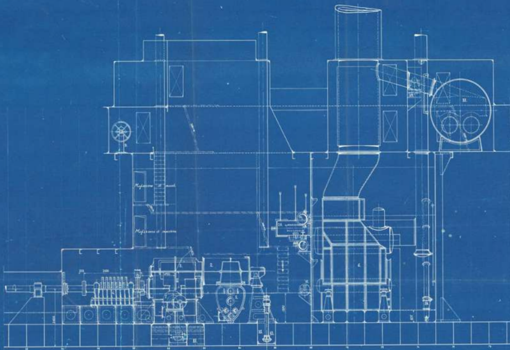
Sezione longitudinale
