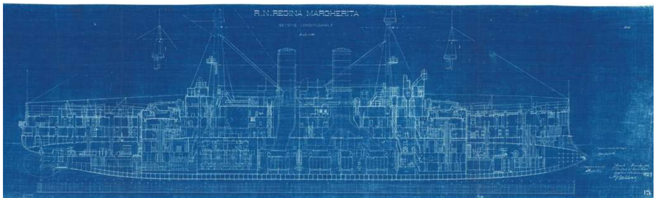
RN Regina Margherita, vista longitudinale, blueprint, Archivio DuilioShip
