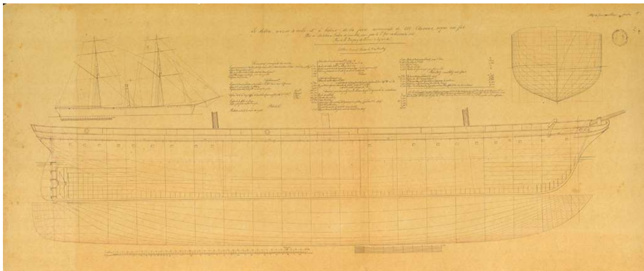
Le Caton, aviso a vela ed elica, Tolone 1848, Atlas 2, Archivio DuilioShip
