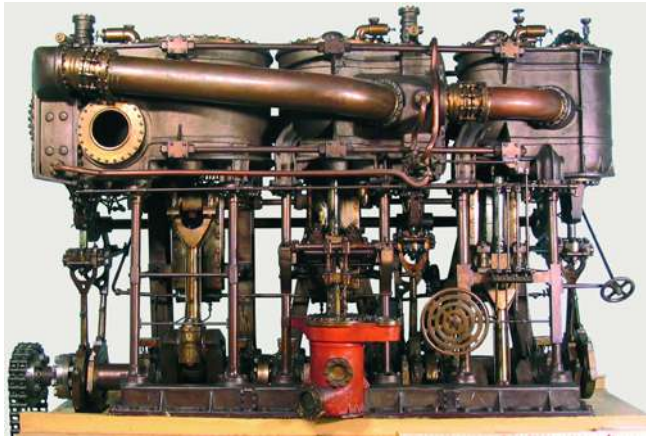
Modello di una delle motrici alternative a vapore verticali facenti parte dell'impianto di propulsione della nave da battaglia corazzata Emanuele Filiberto – Modello didattico conservato dal DITEN
