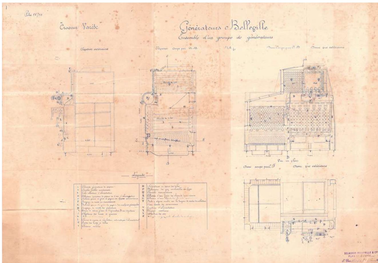
Generatore Delauney Belleville & Co, Ensemble d'un group de générateurs, ciano print seppia, Archivio DuilioShip
