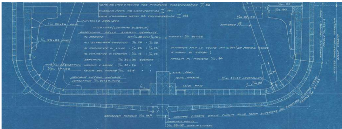
Particolare tratto dal disegno: Piroscalo in legno per trasporto minerale - Modulo di costruzione 3463 Sezione Maestra. Ciano blueprint. Scala 1.25 65 x 63 cm, Archivio DuilioShip
