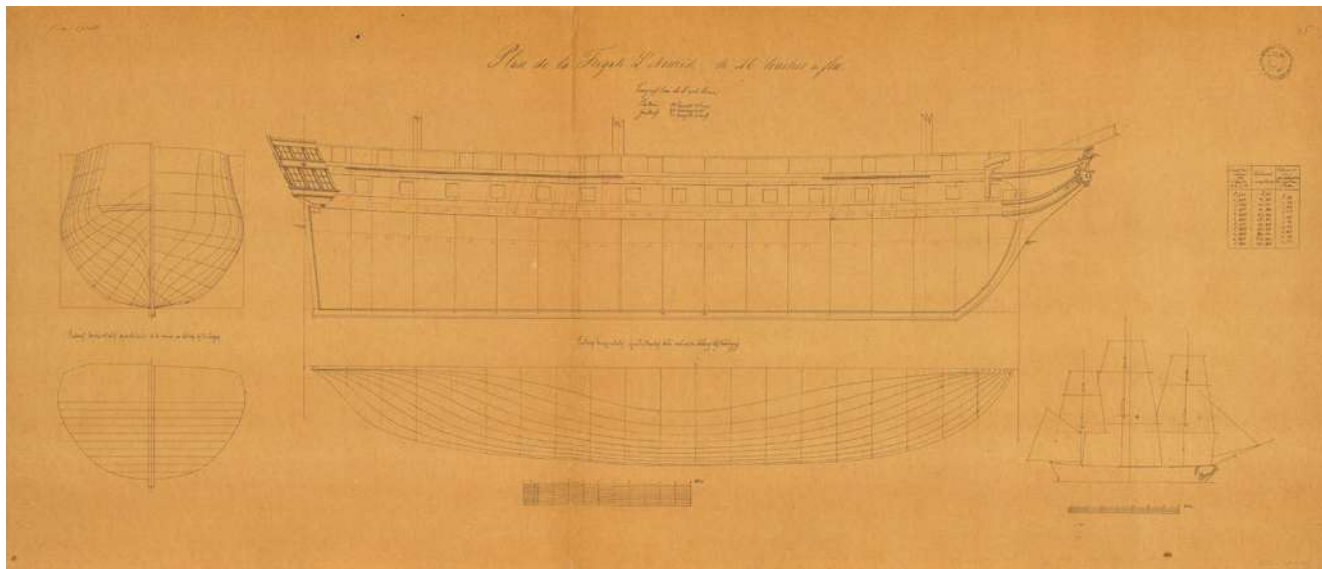
Fregata L'Armide, Tolone 1831, Atlas 1, Archivio DuilioShip
