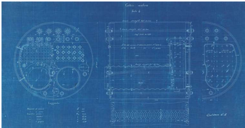
Caldaia ausiliaria cilindrica monofronte a tubi con ritorno di fiamma, blueprint, Archivio DuilioShip
