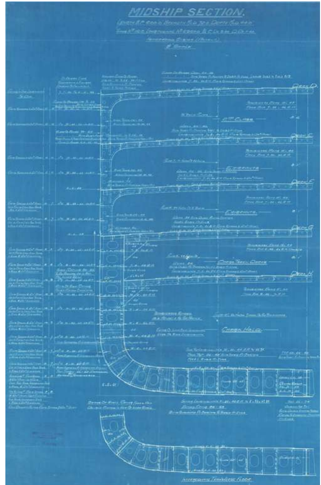
Sezione maestra nave passeggeri a tre eliche, in ferro, metodo Isherwood, Archivio DuilioShip
