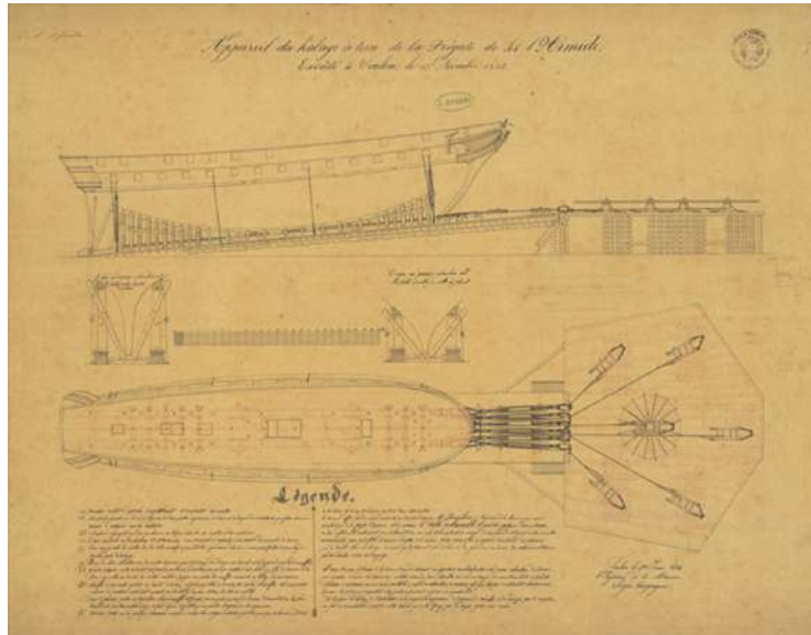
Appareil du halage a terre de la Fregate de 46 l'Armide , litografia su carta velina, Tolone, 1832, raccolta Atlas 1, Archivio DuilioShip
