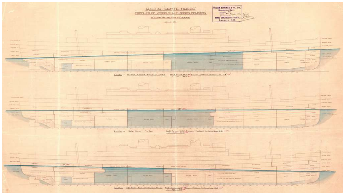
Piroscafo "Conte Rosso", verifica della galleggiabilità di un piroscafo per passeggeri con due compartimenti allagati. g.c. Scuola Politecnica – UniGe, collezione disegni e stampe [478]
