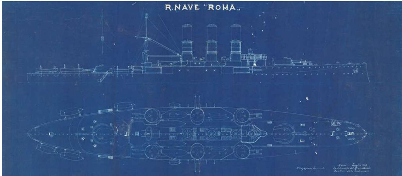
RN Roma, Vista laterale e coperta, blue print, raccolta disegni provenienti da DITEN, Archivio DuilioShip
