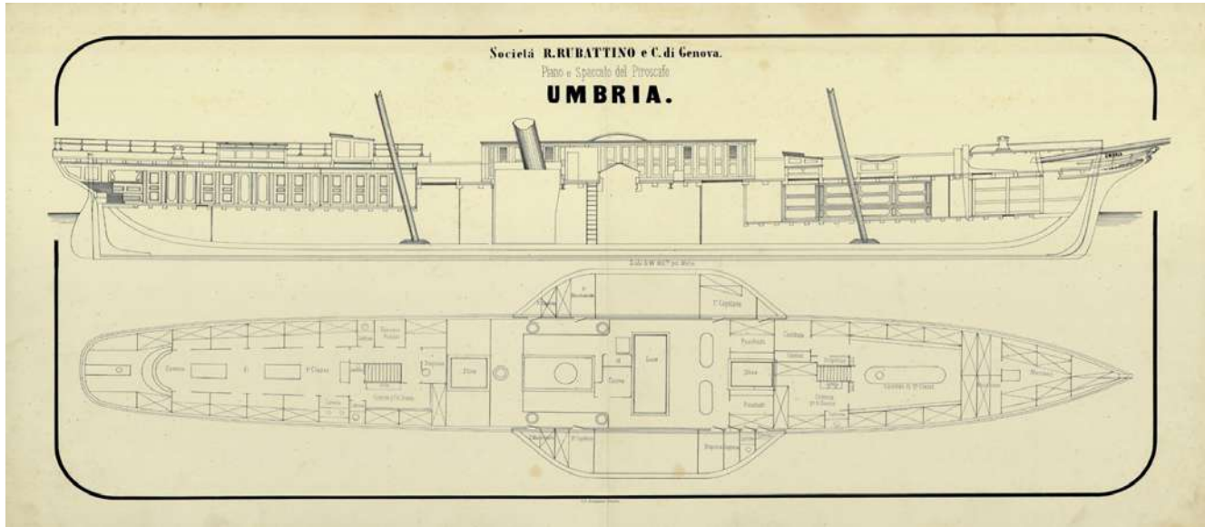
Piroscalo a ruote Umbria. Tavola tratta da «Materiale navale della Società R. Rubattino e C. Concessionari dei servizi postali marittimi», Archivio DuilioShip
