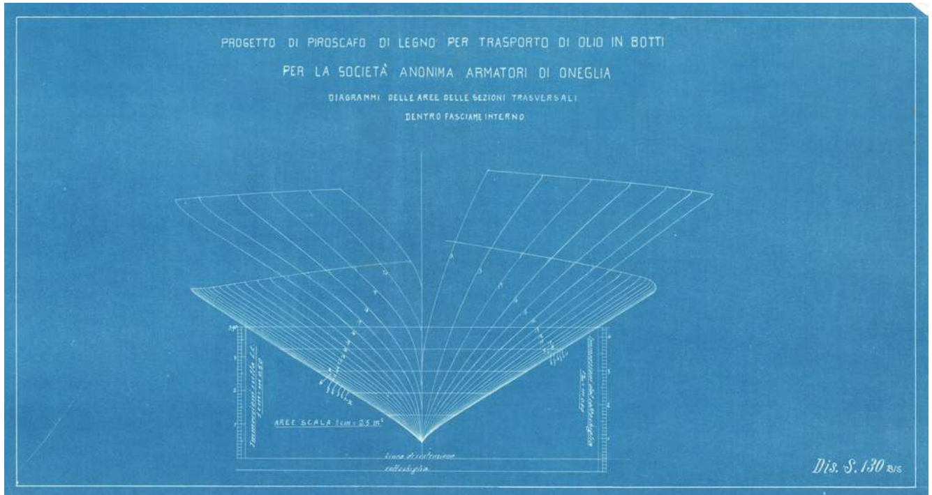
Progetto di piroscavo per trasporto di olio in botti, verticale integrale delle sezioni trasversali
