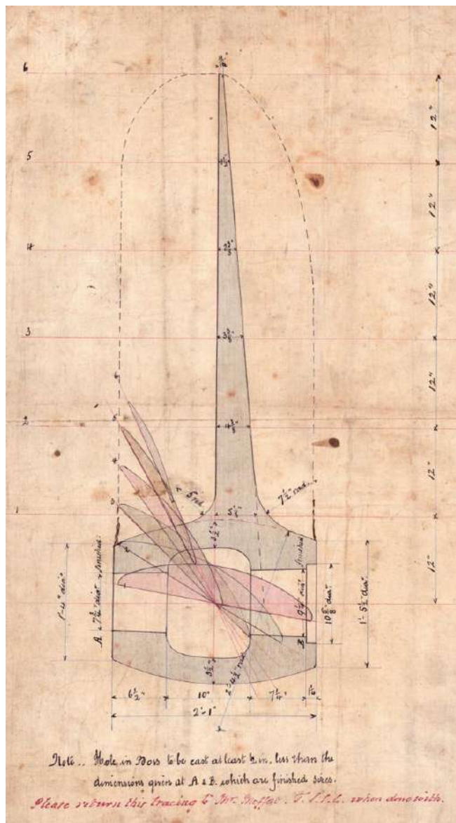
Particolare tratto dal disegno: Screw propeller for the S. S. Warkworth - Disegno a china nero e acquerello su carta lucida. 540 x 360 mm, Archivio DuilioShip
